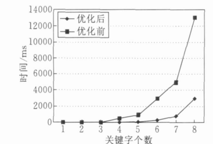
图 6 优化前后模式匹配的时间复杂度
