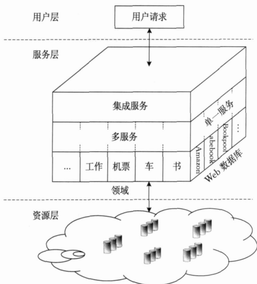
图 1 Deep Web 数据集成服务的基本框架
