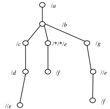
Fig.4 /a/b[c/d//e][g//e/f]/*/*e/f 图 4 /a/b[c/d//e][g//e/f]/*/*e/f
