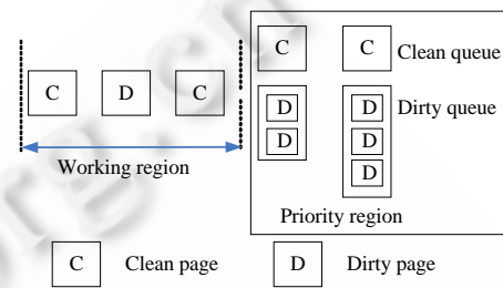
Fig.3 CFDC replacement policy 图 3 CFDC 置换策略示意图
