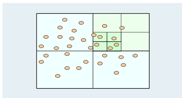
图6 基于四分树的匿名方法
